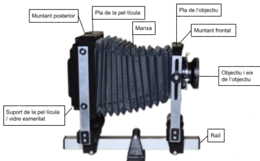
Figura 56. Parts de la càmera de gran format. (2023)
